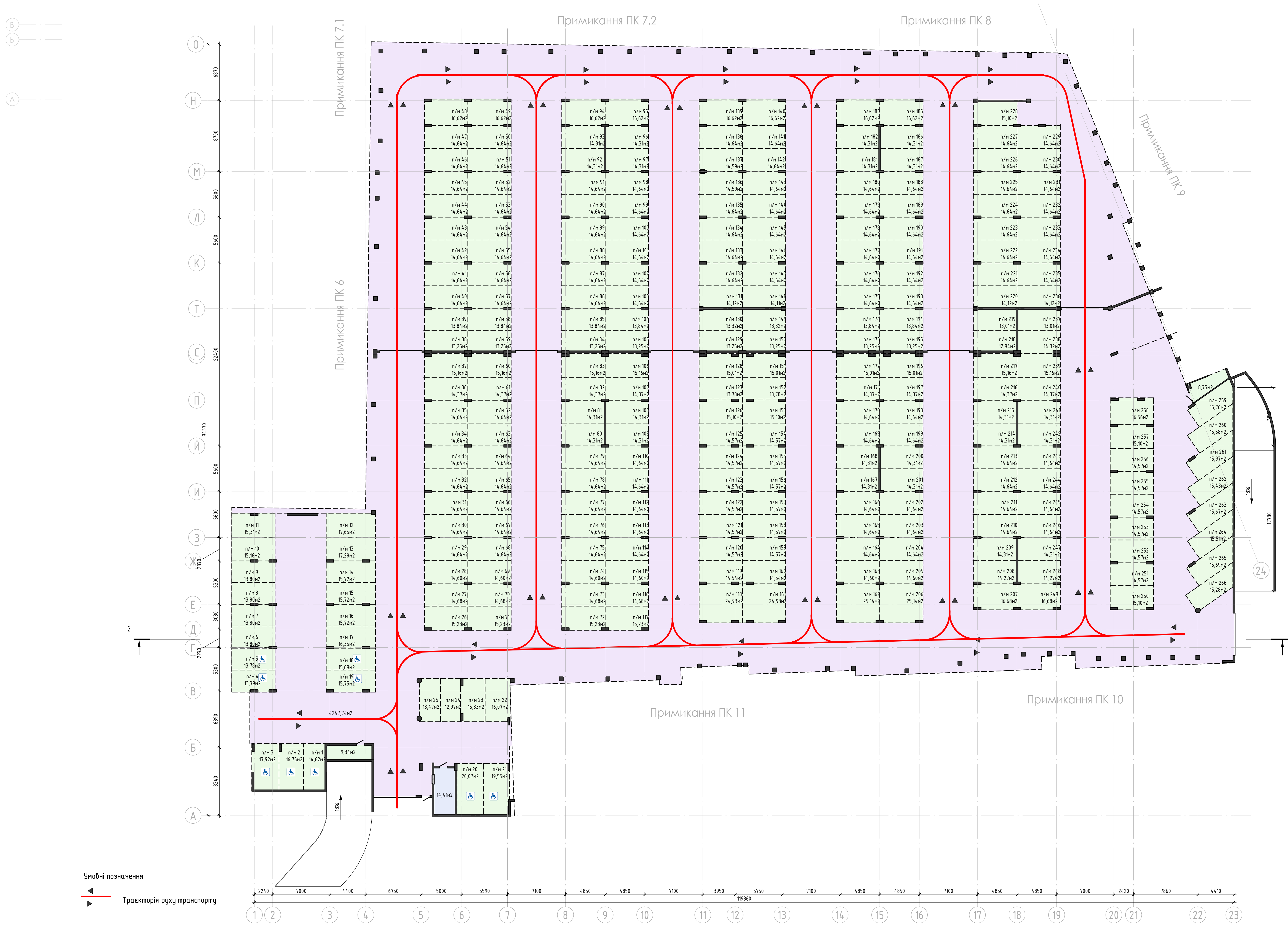
План паркінгу на відмі -0.400 (1 : 200)
