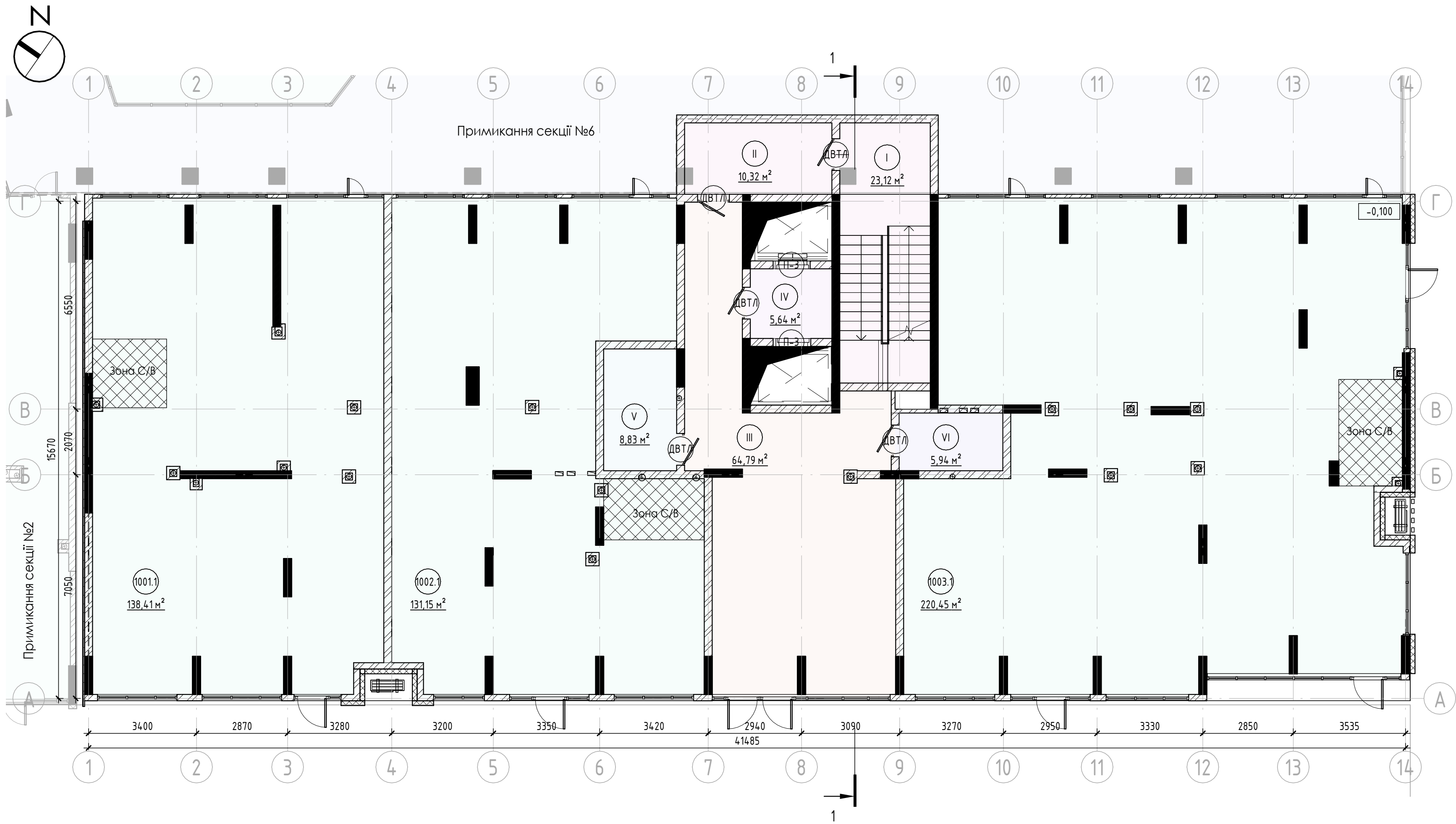
Схема розташування секцій ЖК
