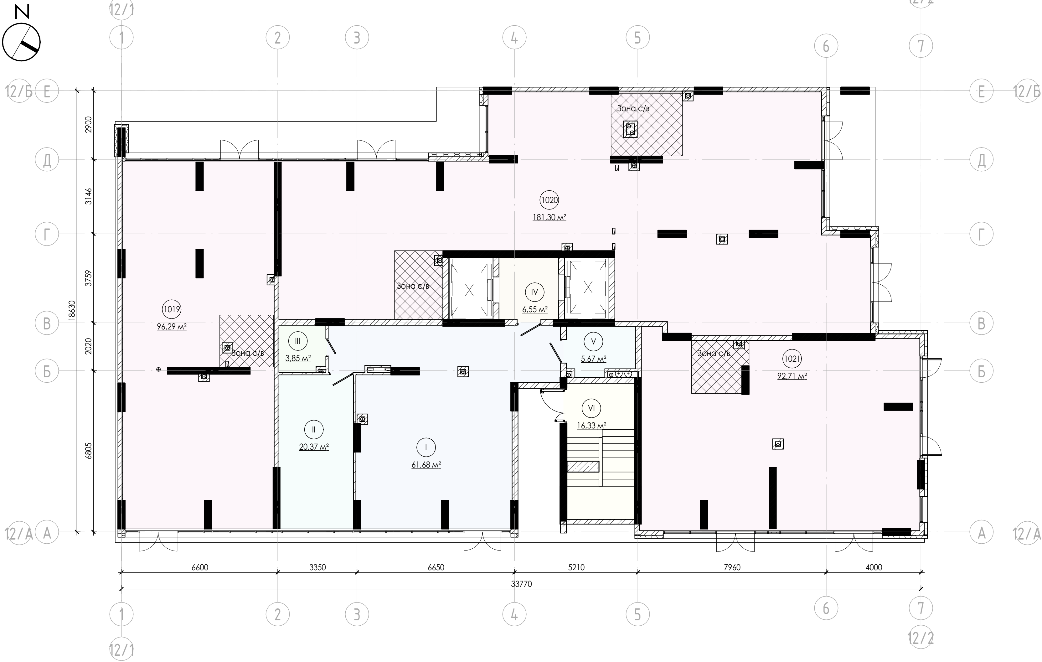
Експлікація приміщень 1-го поверху
